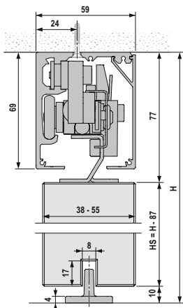
Deckenmontage
