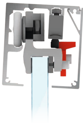
Aktivator unten
