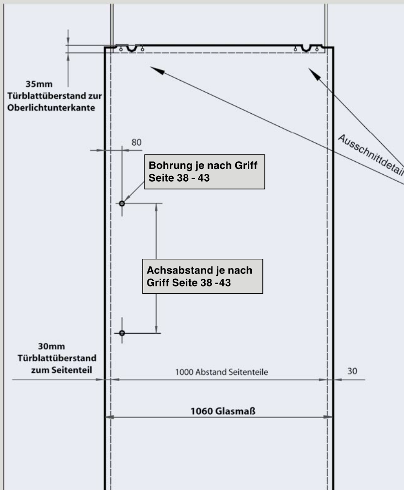
Glasausschnitt DETAIL Z, für Rollenwagen System Habicht
