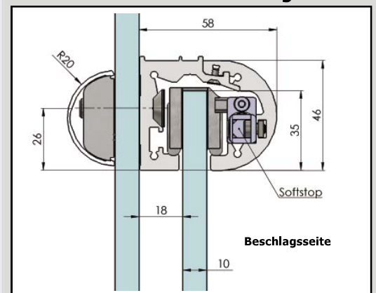
Schnittansicht Glasanbindung
