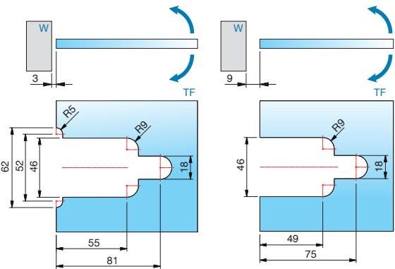
Glasbearbeitungen für die unterschiedlichen Spaltmaße
