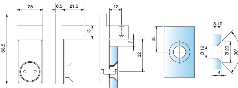
beidseitig 90° verstellbar 8474MS7/MS10/MSPVD22 verschiedene Längen, siehe Seite 208
