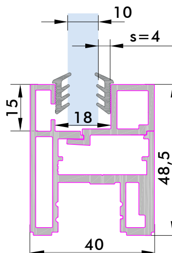
ESG 10 mm
