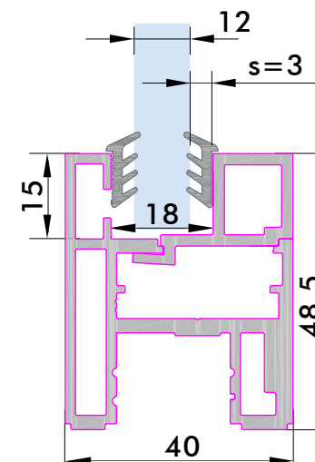
ESG 12 mm
