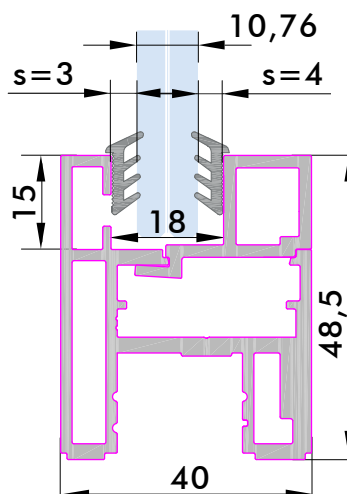
VSG 10,76 mm
