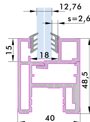
VSG 12,76 mm
