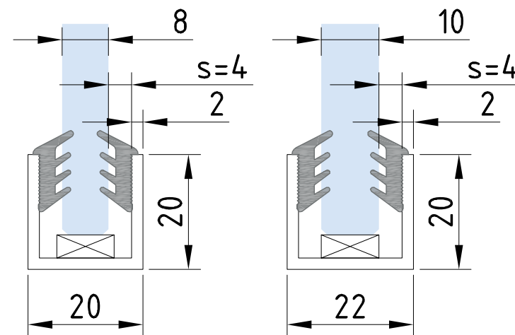
Einbausituation 608613; s= 4 mm
