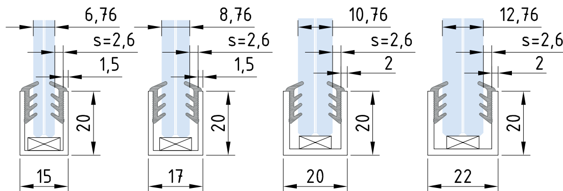
Einbausituation 608611; s= 2,5 - 2,6 mm
