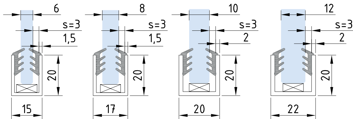
Einbausituation 608612; s= 3 mm
