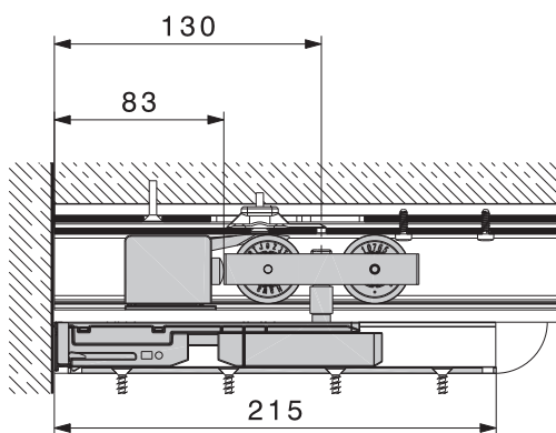
Türposition: geschlossen
