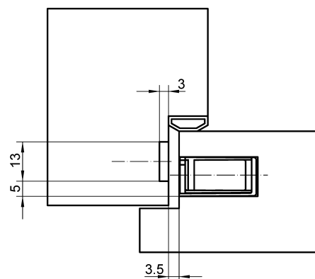
Querschnitt 2
