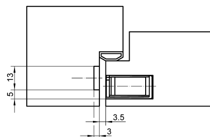
Querschnitt 3
