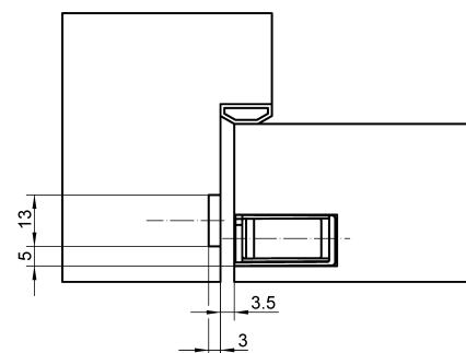
Querschnitt 1
