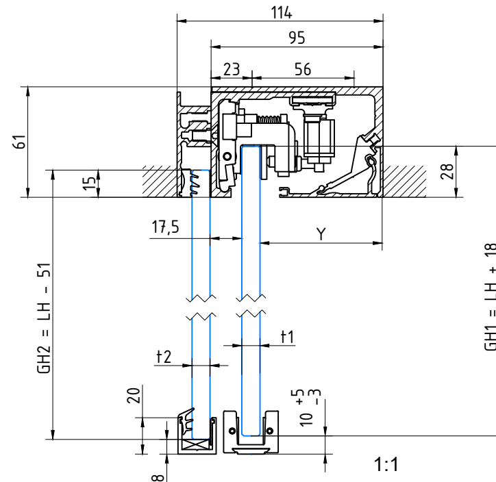
Art. Nr. 36.276 Montage in Decke mit Seitenteilen
