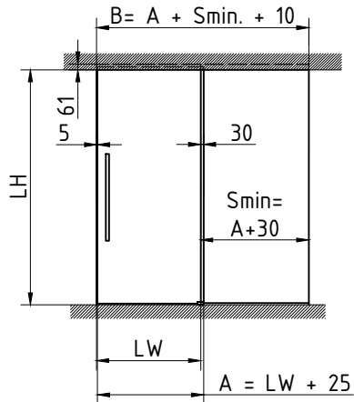
Art. Nr. 36.243 Montage in Decke mit Seitenteil
