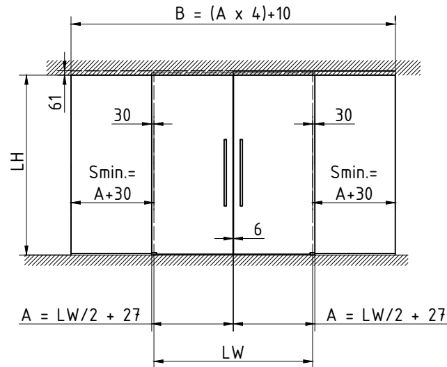
Art. Nr. 36.244 Montage in Decke mit Seitenteilen
