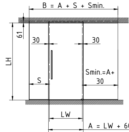
Art. Nr. 36.276 Montage in Decke mit Seitenteilen
