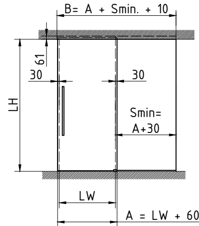
Art. Nr. 36.275 Montage in Decke mit Seitenteil
