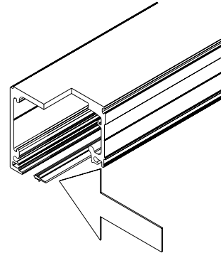
Laufschiene mit Sichtschutzprofil
