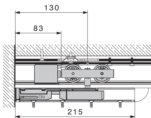
Türposition: geschlossen
