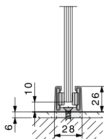
Spielfreie Bodenführung
