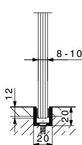
U-Profil mit Gleitelemente
