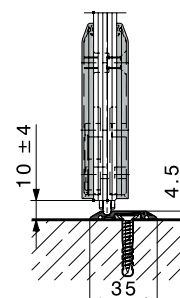
Einfachführungsschiene
