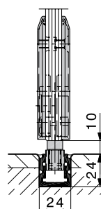
Führungsschiene
