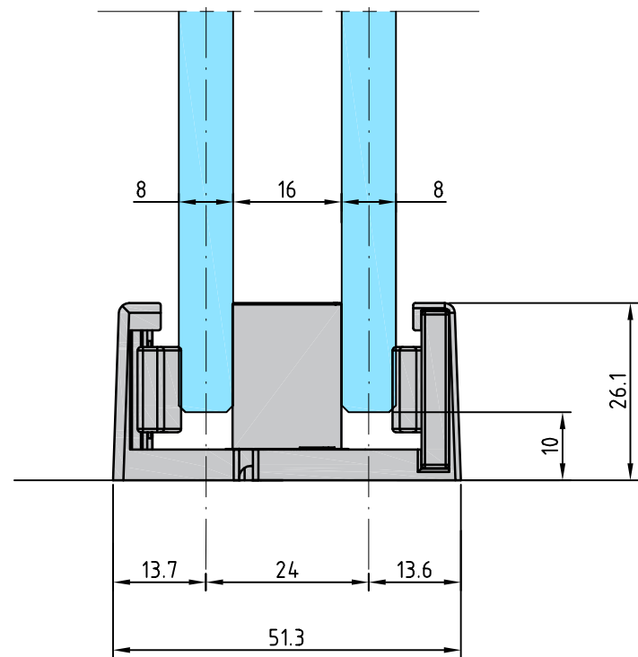
19138 HAWA Bodenführung für ESG 8 mm
