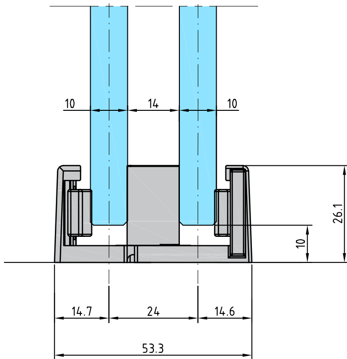
19138 HAWA Bodenführung für ESG 10 mm
