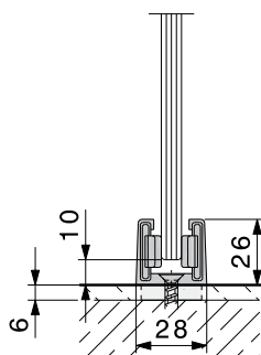
Bodenführungsvarianten
