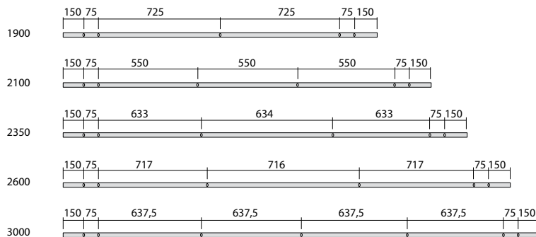
Bohrmaß
