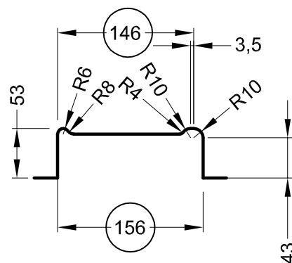
Unica Detail Y
