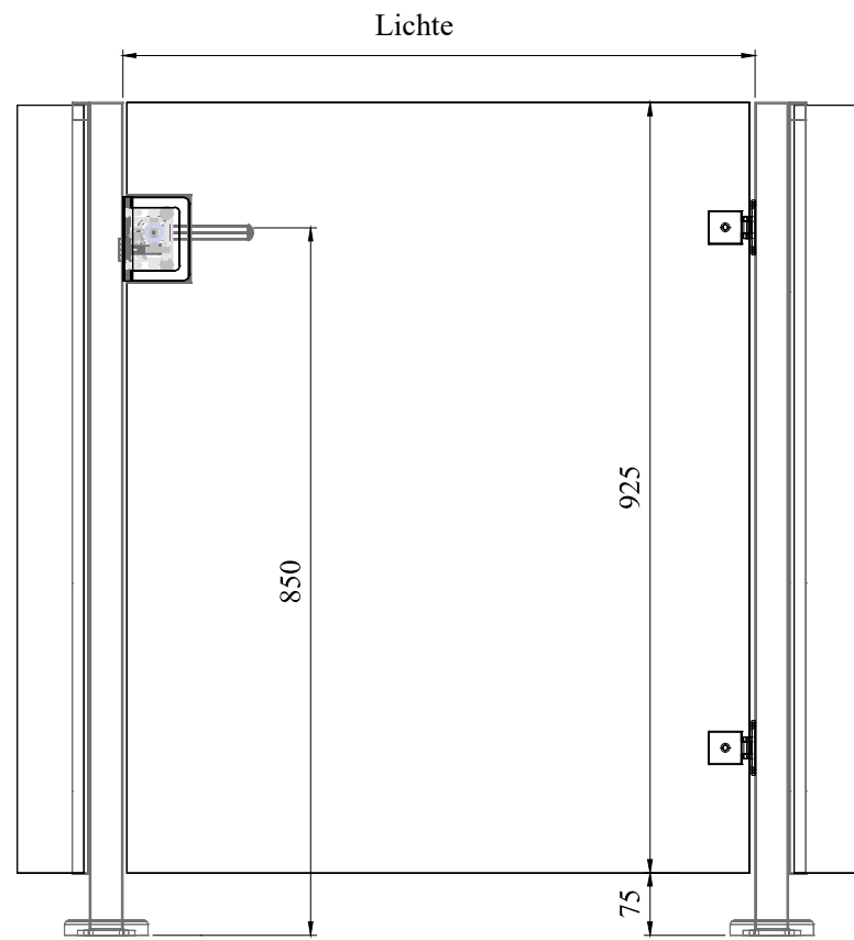
Aufriss
