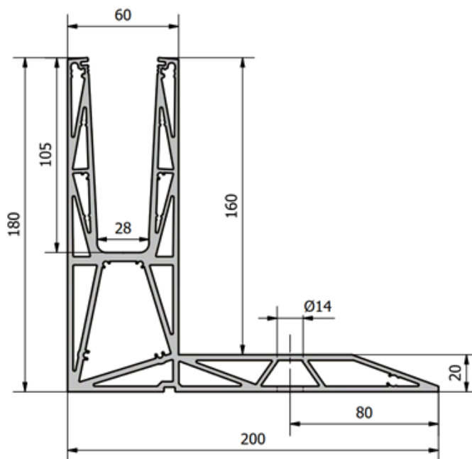
TL-3120
