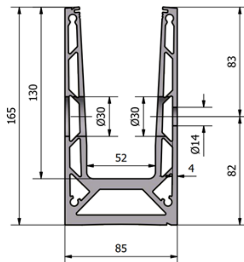
TL-6041
