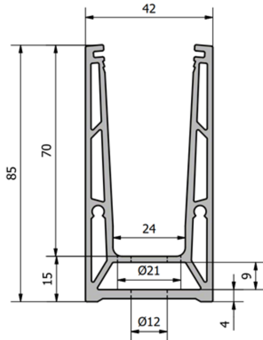
TL-6500
